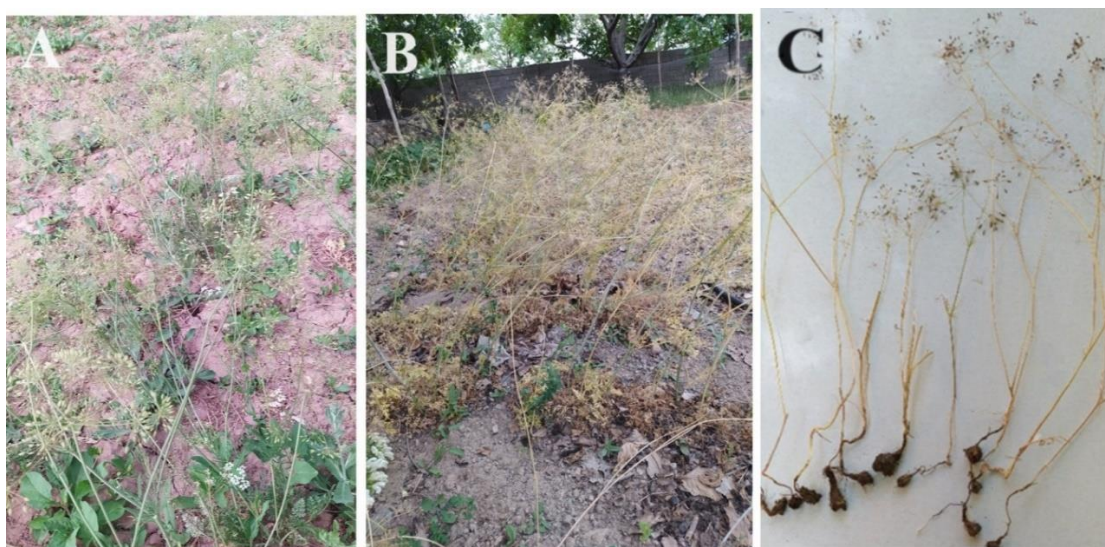
شکل ۶. تشکیل میوه در زیره سیاه در سال چهارم ( B. persicum )، A و B، به ترتیب در ساردوئییه و مزرعه دانشگاه شهید باهنر کرمان، C. بخش زیرزمینی چوب‌پنبه‌ای شده.
